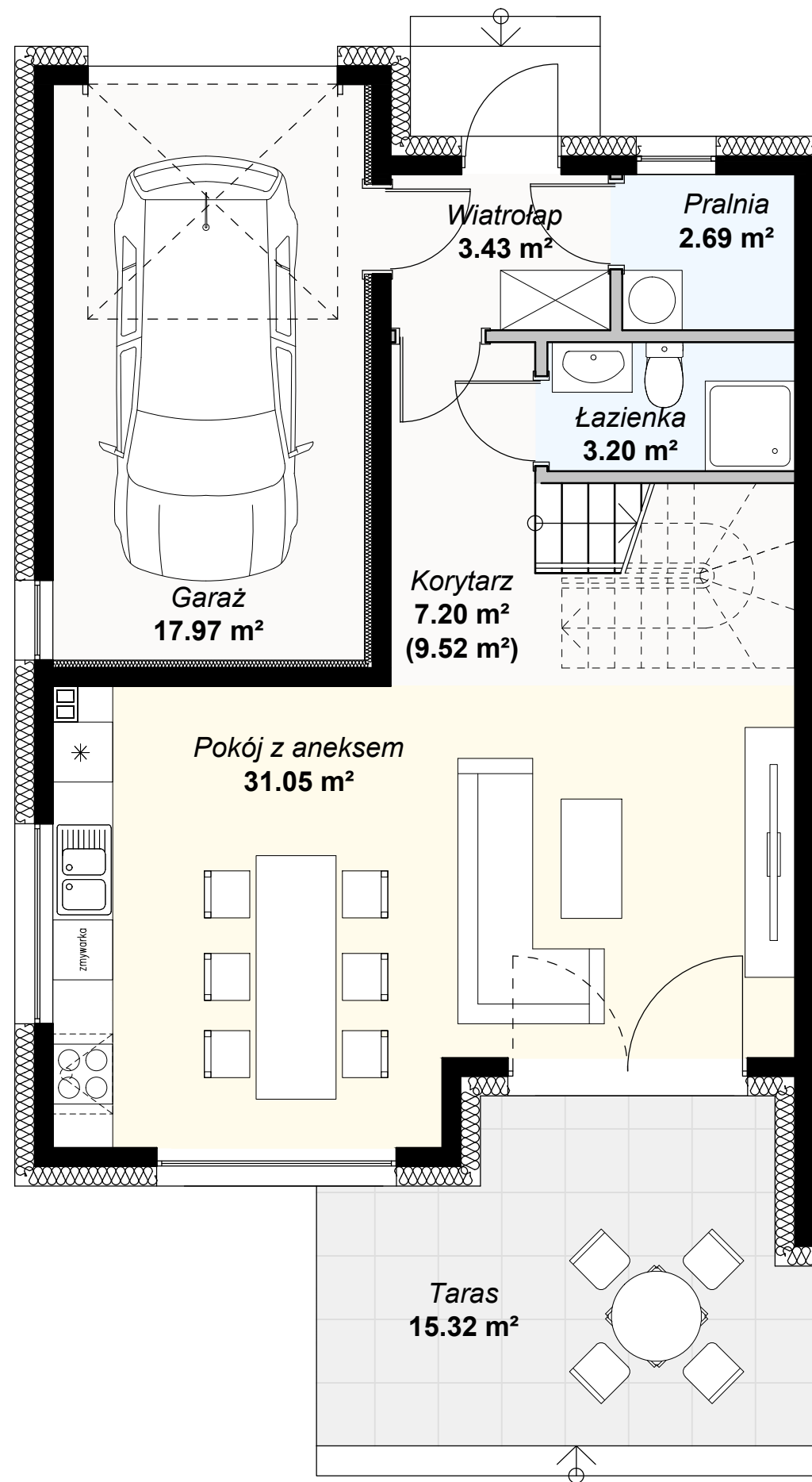
rzut parteru
