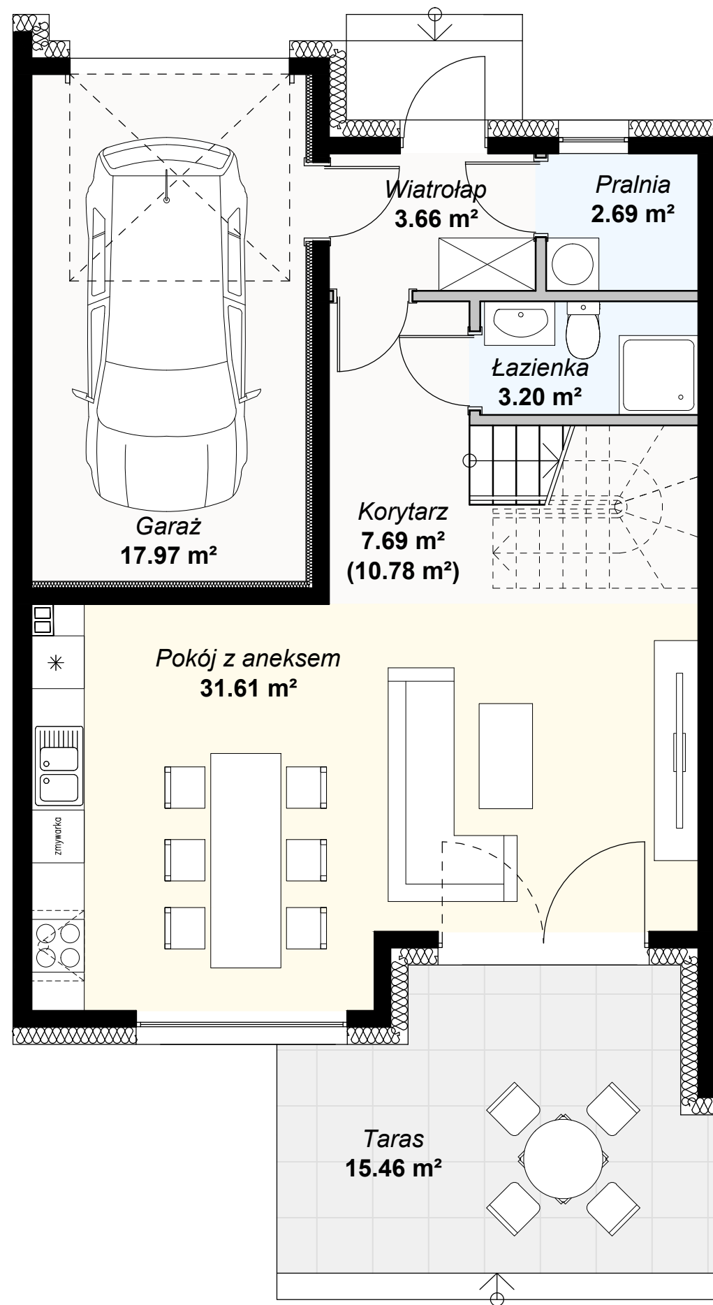
rzut parteru
